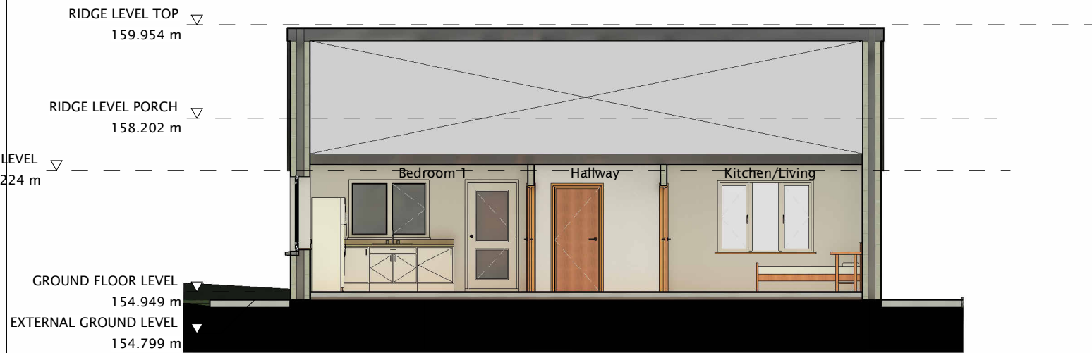
1 Long Section 1 : 100
