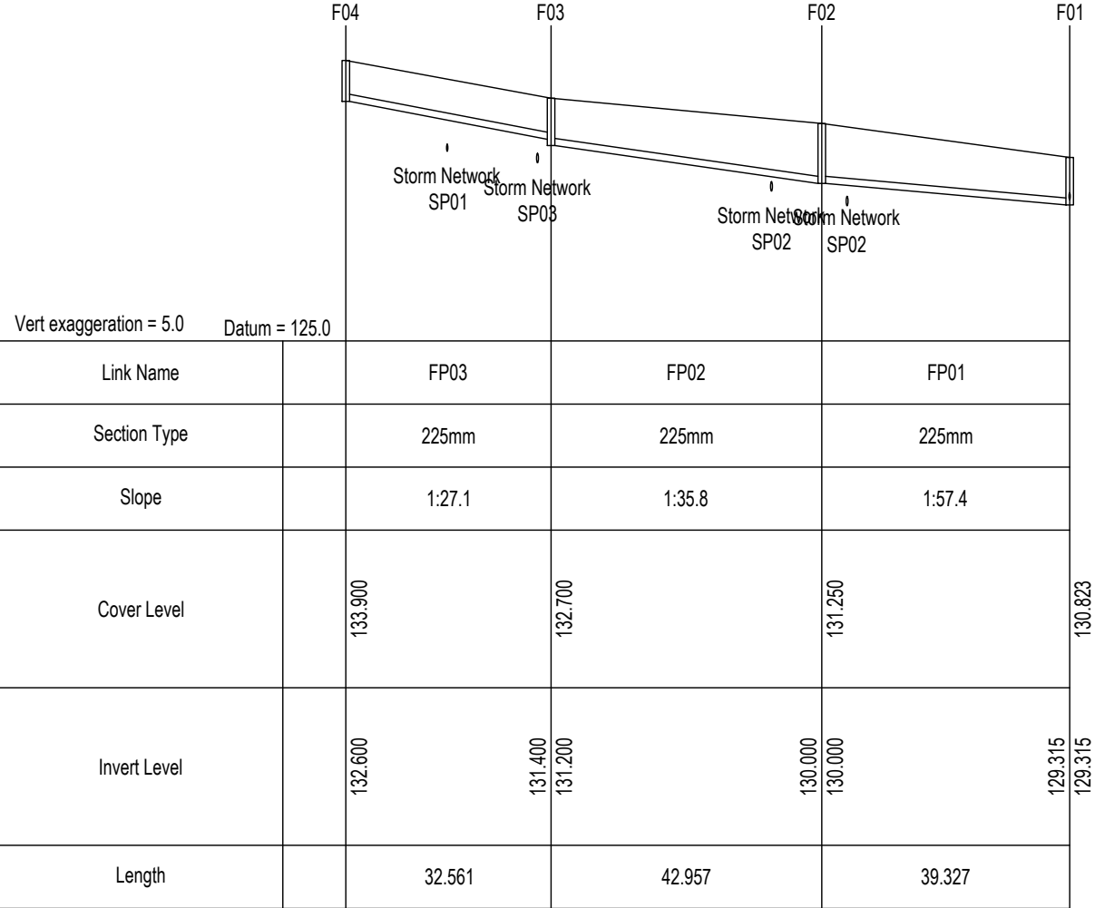
FOUL SEWER LONGITUDINAL SECTION Scale 1:1000 / 1:200
